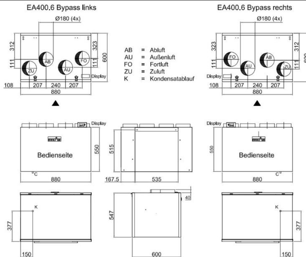
Fig. 6 Maßskizzen EuroAir 400 (mit internen Bypass, rechte Ausführung)
